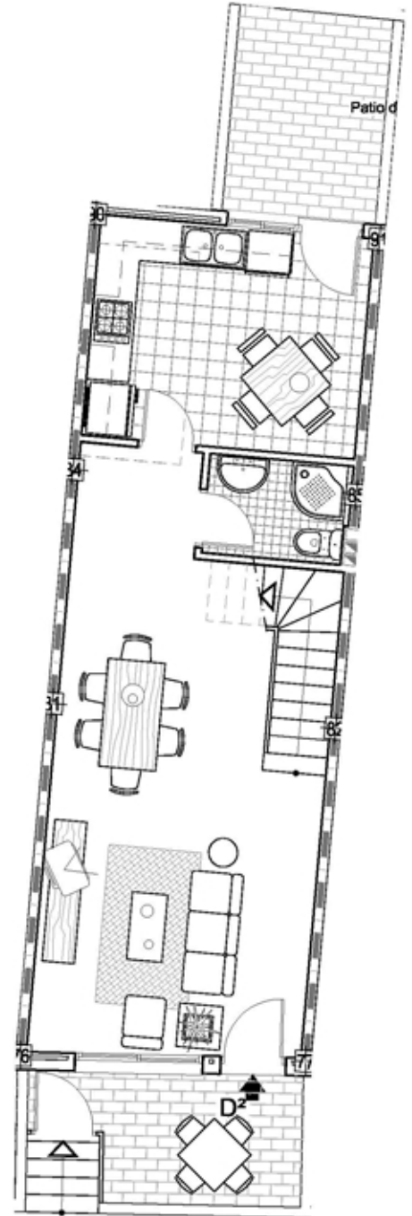
PLANTA BAJA
